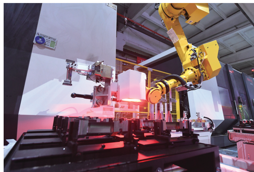
哈电汽轮机中小叶片自动加工生产线机械手臂正在装卡叶片。
